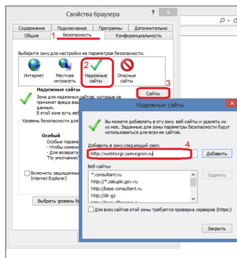
Рисунок 3 - Добавление адреса Портала в список надежных узлов
