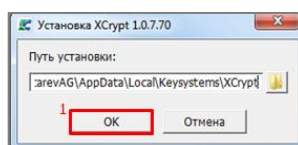
Рисунок 11– Установка XCrypt
