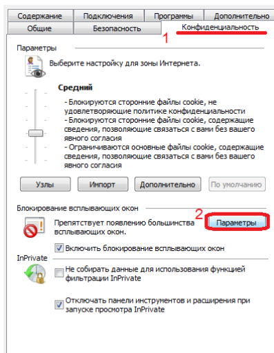
Рисунок 4 - Вкладка Конфиденциальность
